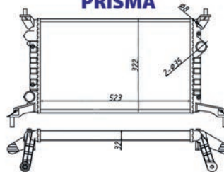
RADIADOR C/AR (MANUAL) 29819 - RF
