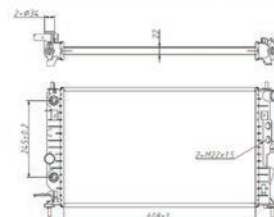
RADIADOR C/AR (AUTOMATICO) 29805 - RF
