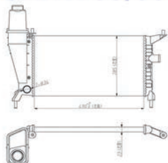
RADIADOR S/AR C/RESERVATORIO (MANUAL) 29812 - RF
