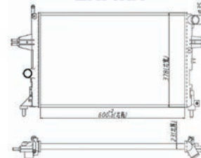
RADIADOR S/AR (MANUAL) 29813 - RF
