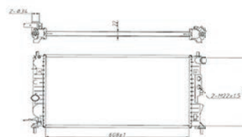
RADIADOR C/AR (AUTOMATICO) 29804 - RF
