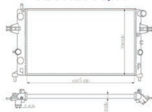
RADIADOR C/AR (MANUAL) 29814 - RF
