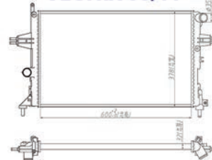
RADIADOR C/AR AUTOMATICO 29815 - RF
